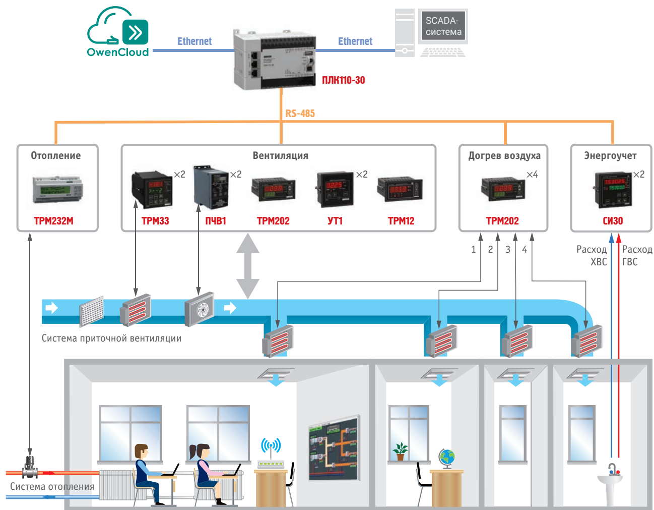
Рис. 1. Система диспетчеризации
