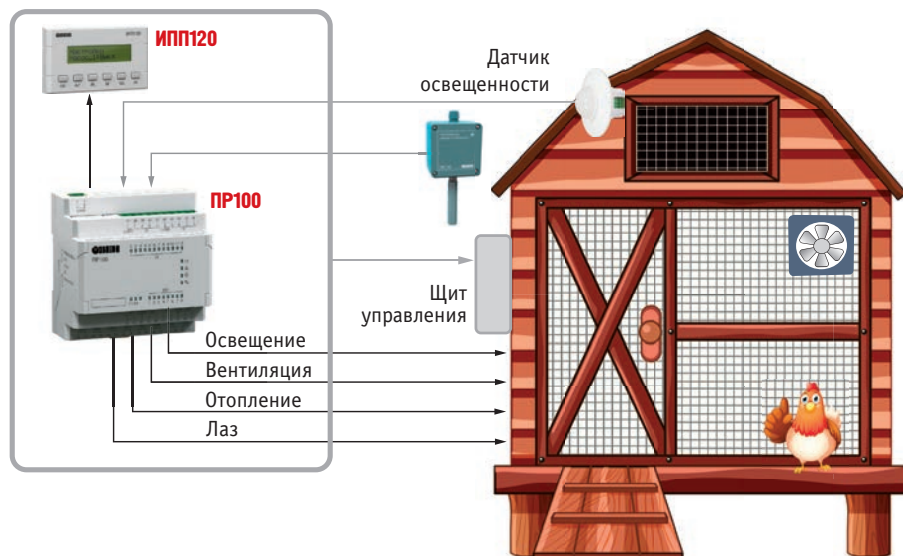
Рис. 1. Система управления на базе OWEN PR100
