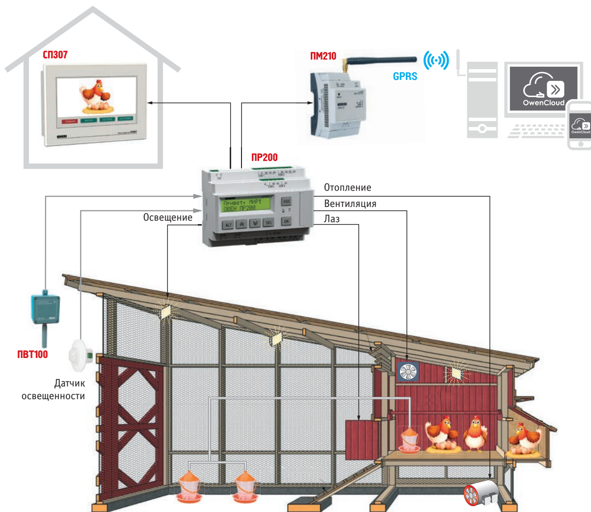
Рис. 2. Система управления на базе OWEN PR200
